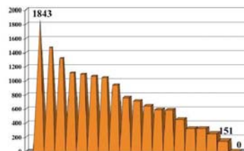
15 座锥型海山水深不足 2 500 米部分的总表面积
