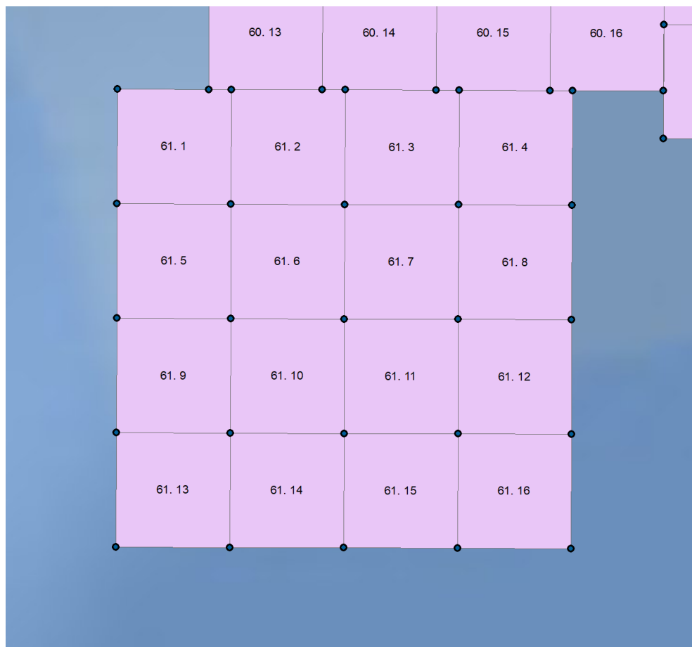
Рисунок 2 Разбивка блока кобальтоносных железомарганцевых корок на 16 равных клеток размером 1,12 × 1,12 км и индексация этих клеток
