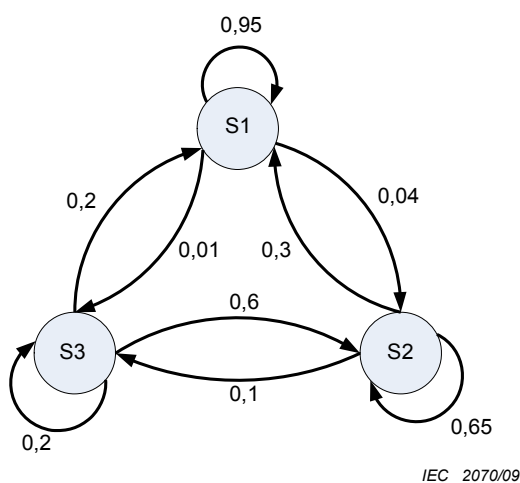
Figure B.9 – Exemple de diagramme de Markov du système
